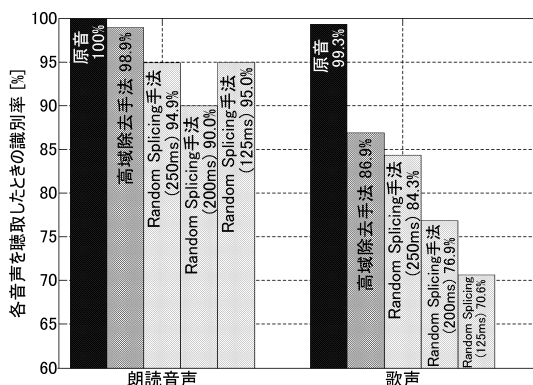
図3 Random Splicing，高域除去した音声信号の識別率
