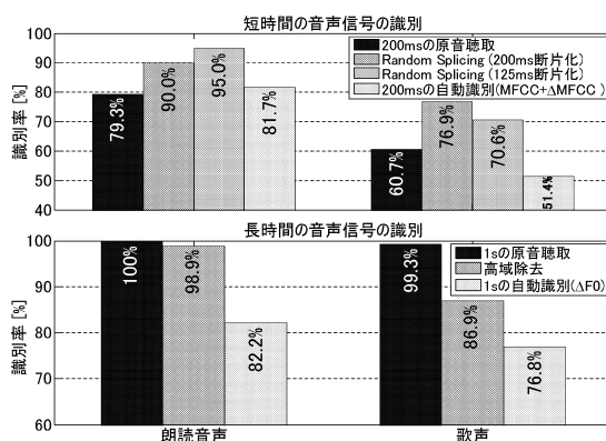
図10 聴取実験結果と自動識別手法の性能との比較
