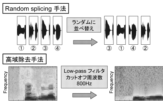
図2 Random splicing 手法と高域除去手法
