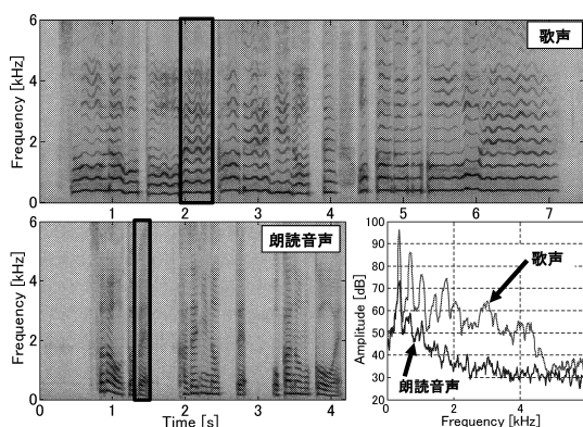
図4 歌声と朗読音声のスペクトログラム（同一歌詞を発声）
