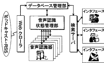
図 3: PodCastle のシステム構成図
