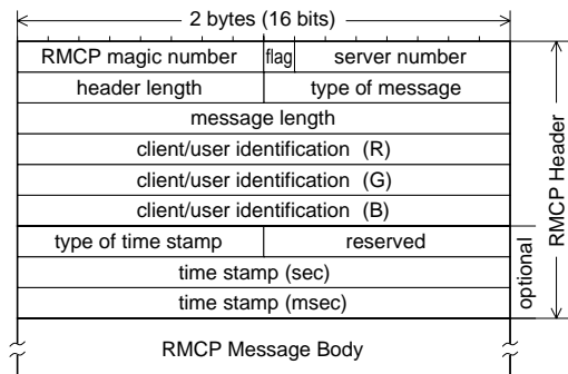
図 2: RMCP パケットの構造
