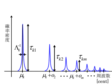
図 1 単一基底に対する混合ガウス分布
