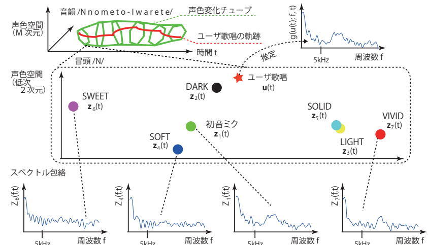
図5 声色空間における各点には、スペクトル包絡がそれぞれ対応付けられており、ユーザ歌唱がその点に重なった時は同じスペクトル包絡が生成されるように補間する。ここでは、実際に構成した声色空間上のある時刻における初音ミクと初音ミク・アペンド (DARK, LIGHT, SOFT, SOLID, SWEET, VIVID) の配置を示す。
