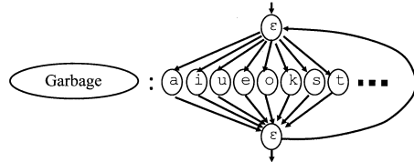
図4 ガベージモデル (HMM)。
